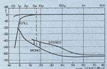
UKW-Frequenzgang und UKW-Übersprechdämpfung: auch bei hohen Frequenzen breiteste Stereo-Wirkung.
