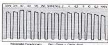
Wiedergabe-Frequenzgang Chrom-Band.
