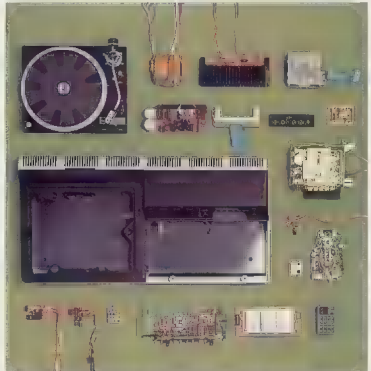
Alle Geräte des Blaupunkt HiFi-Systems Digita 500 sind moduliert. Ihr Vorteil: Die einzelnen Baugruppen lassen sich leicht und schnell austauschen.
