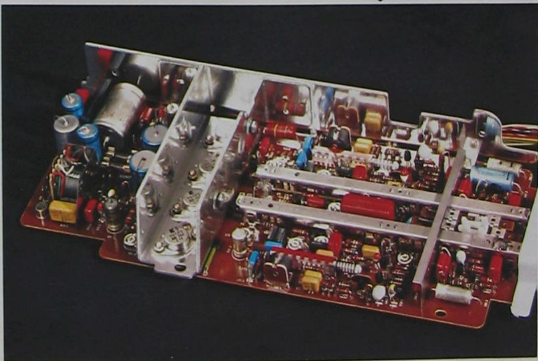
Das ist die Verstärkerplatte vom TK 248 HI-FI: modernste Technik klar und übersichtlich aufgebaut.
