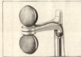
Mikrofon GDSM 200 Mit Anschlußkabelpaar 4 m und Schnurübertragern • Stativgewinde • Für hochwertige Stereoaufnahmen, auch in akustisch nicht vorbereiteten Räumen • Ausgezeichnete Richtcharakteristik • Frequenzbereich: 100...16000 Hz. DM 195,-
