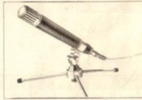
Mikrofon GDM 322 Für Sprach- und spezielle Orchesteraufnahmen auch bei ungünstigen Raumverhältnissen • Mit Tischstativ und Stativanschlußteil • Nierencharakteristik • Frequenzbereich: 50...17000 Hz. DM 110,-
