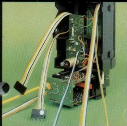
Die zukunftsweisende elektronische Perfektion der Loewe-Stationspeicherung von innen.
