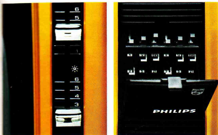
Komfort-Bedienfeld mit 3 Schiebepfeilern für Lautstärke, Helligkeit, Kontrast und 6 Programm-Tasten für schnelle Programmwahl.
