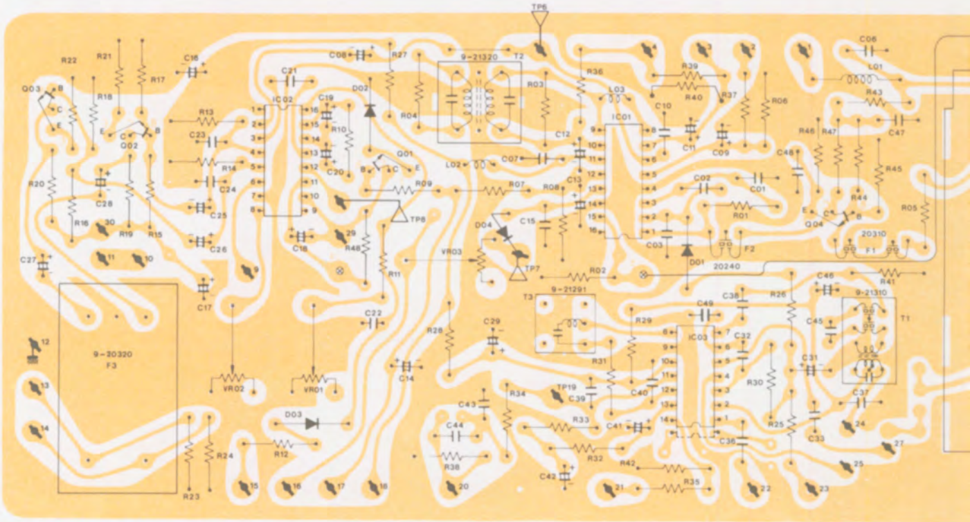
PLATINE HF-FI (côté éléments)
