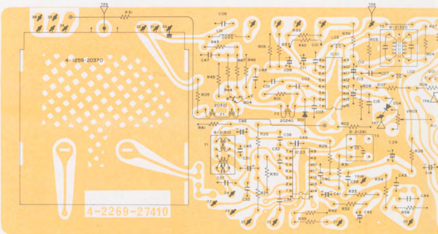
PLATINE HF-FI (côté cuivre)
