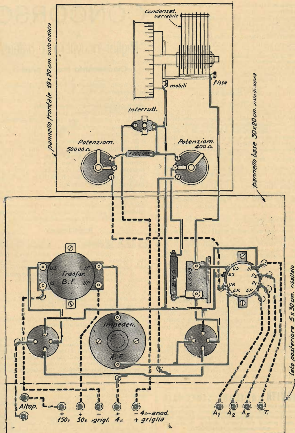
Schema costruttivo del « Simplex »
