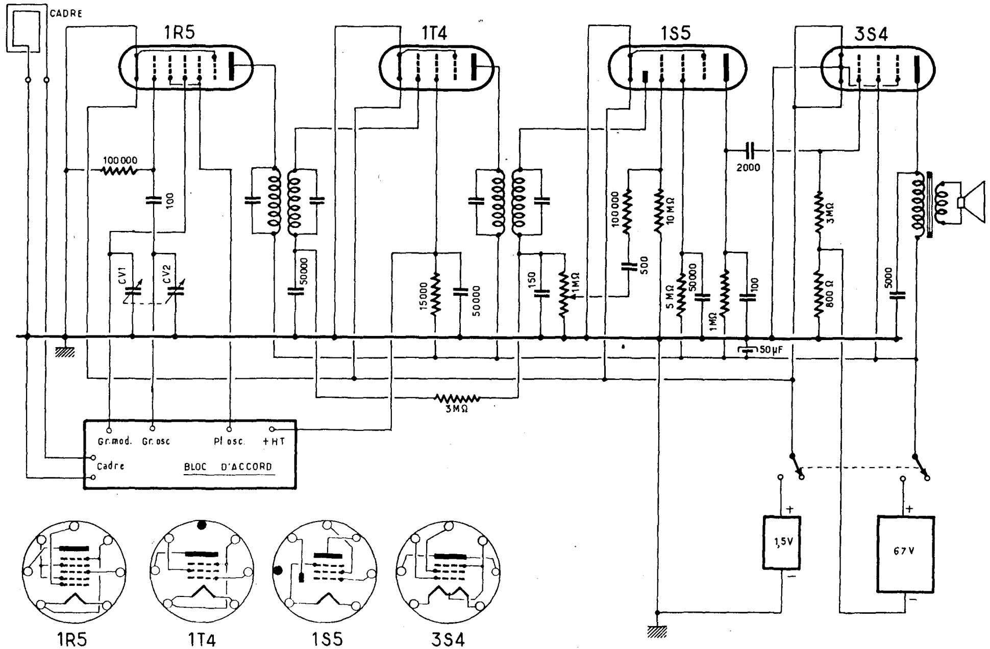
Schéma général commun aux récepteurs P4 et PP4.
