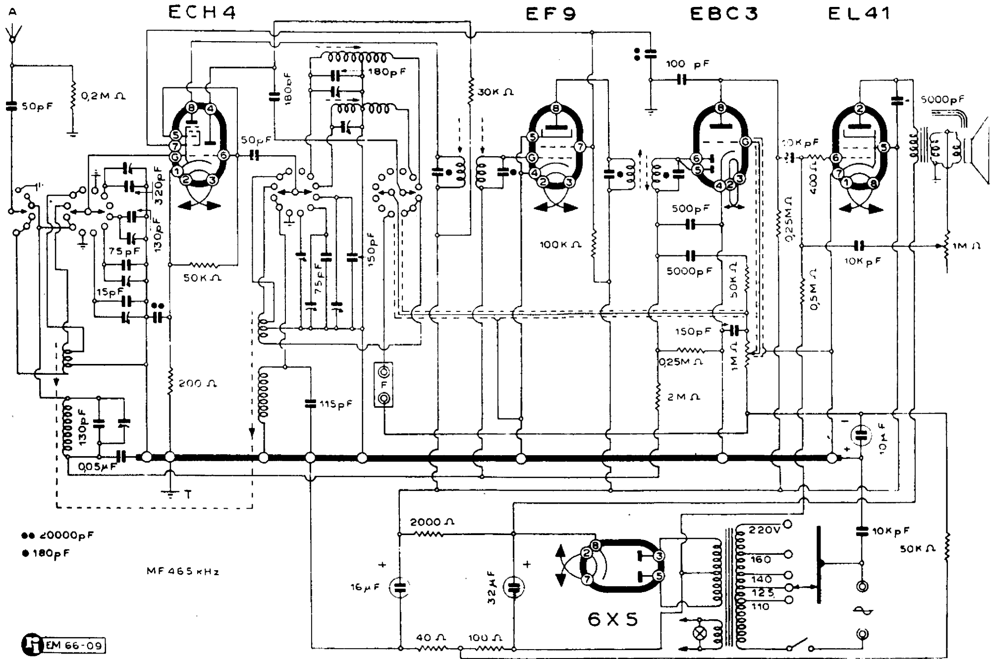
A.B.C. RADIOCOSTRUZIONI - Mod. R 951/F - R 951/F
