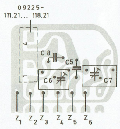
Zwischenkreis INTERMEDIATE CIRCUIT CIRCUIT INTERMEDIAIRE CIRCUITO INTERMEDIO
