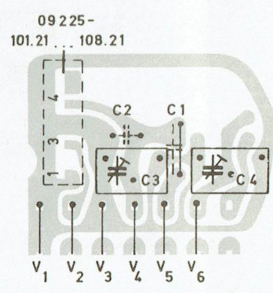
Vorkreis INPUT CIRCUIT CIRCUIT D'ENTREE PRESTADIO
