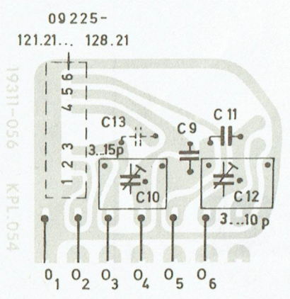
Oszillatorkreis OSCILLATOR CIRCUIT CIRCUIT D'OSCILLATEUR CIRCUITO OSCILLATORE
