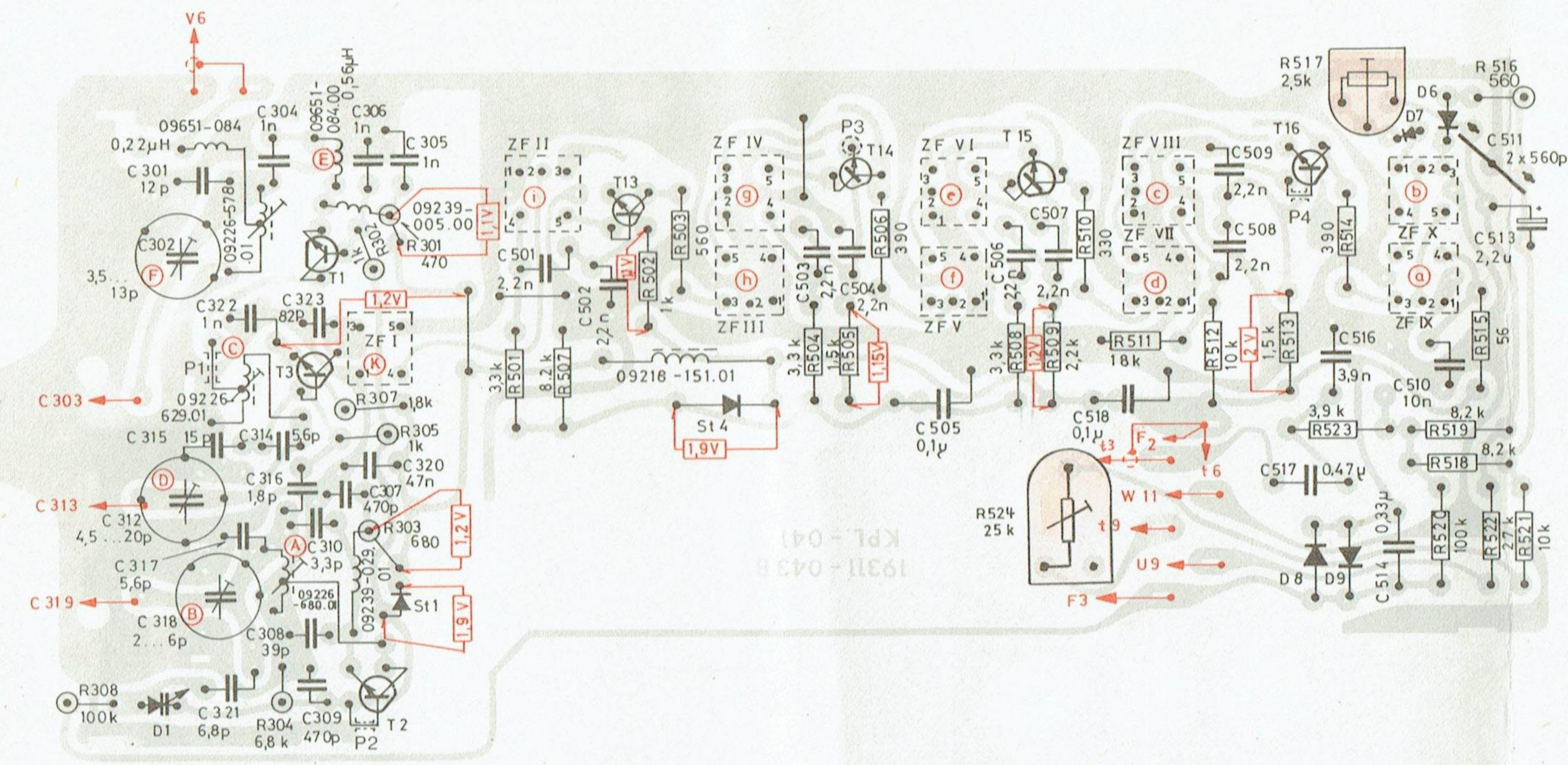
FM-Platte, Lötseite FM-PRINTED BOARD, SOLDER SIDE PLAQUE-FM, VUE DU COTE DES SOUDURES PIASTRA-FM, LATO SALDATURE
