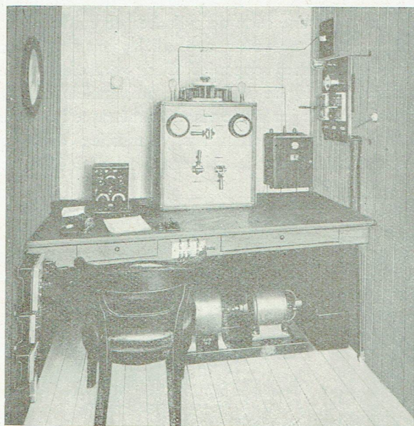
Poste de bord de la Société Indépendante de T.S.F. (fig. 6.)
