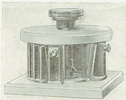
Éclateur " Société Indépendante de T.S.F. "
