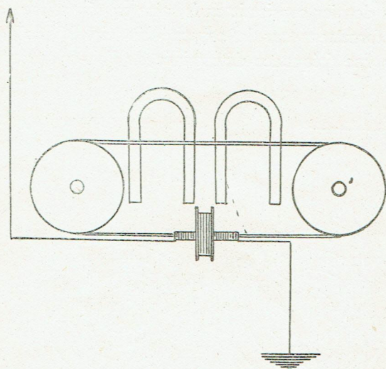
Détecteur Magnétique Marconi.
