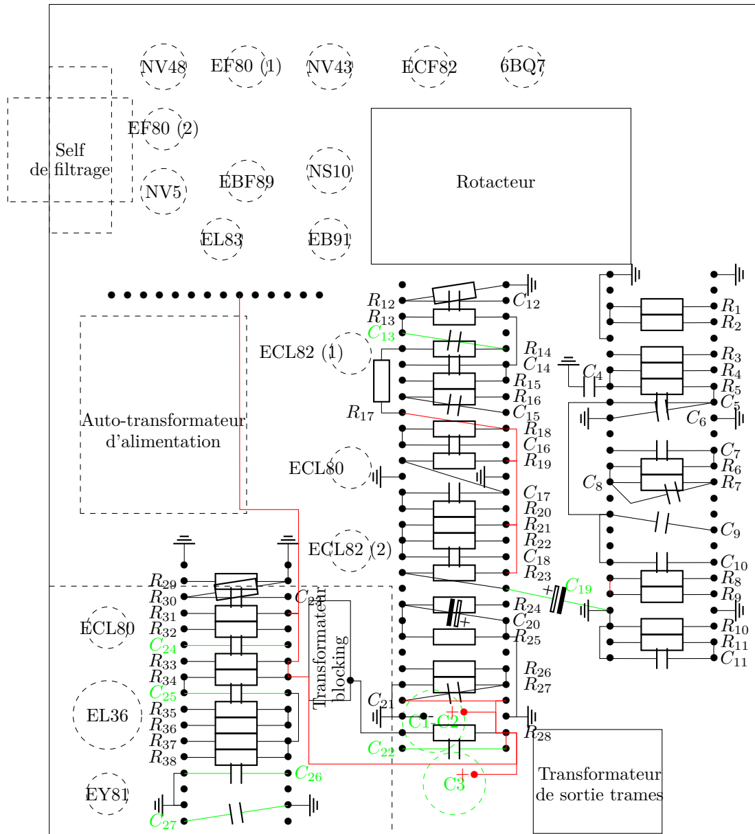
Figure 1: Châssis du téléviseur SNR (vue de dessous)
