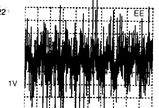
A: AC, 500mV/Div, 1ms/Div IC 7205 Pin 2
