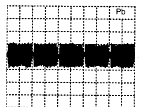
A: AC, 200mV/Div, 10ms/Div IC 7004 Pin 46
