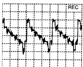
A: AC, 100mV/Div, 20us/Div IC 7004 Pin 40
