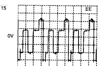
A: AC, 10 V/Div, 20us/Div Transistor 7187 Emitter
