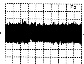
A: AC, 200mV/Div, 5ms/Div IC 7007 Pin 20
