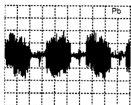
A: AC, 100mV/Div, 20us/Div IC 7004 Pin 52
