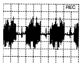
A: AC, 100mV/Div, 20us/Div IC 7004 Pin 52
