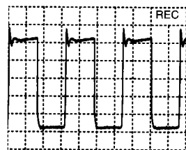
A: AC, 10 V/Div, 20us/Div Transistor 7501 C
