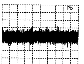
A: AC, 100mV/Div, 100us/Div IC 7072 Pin 13
