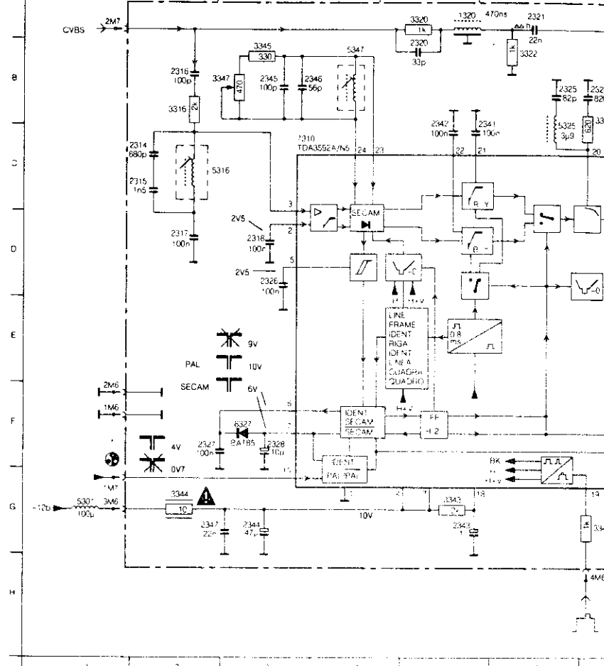
1020 SECAM/PAL TRANSCODER/TRANSCODIFICATORE
