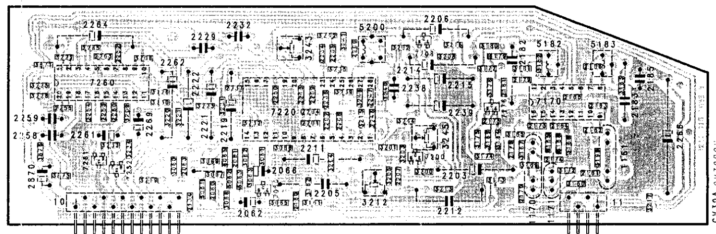
1995 STEREO SOUND MODULE
