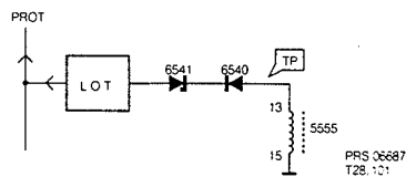
Die Amplitude des Rücklaufimpulses steigt, wenn z.B. der Rücklaufimpuls wegen eines Fehlers in der Leitungsendstufe verkürzt wird. Dadurch wird über die durchgeschaltete Z-Diode D6541 die Schutzschaltung aktiviert.
