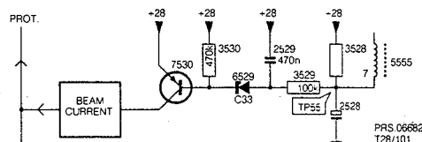
Bei einem zu starken Anstieg des Strahlstroms sinkt die Spannung über C2528 ab, so dass die Z-Diode D6529 durchschaltet und über TS7530 die Schutzschaltung aktiviert wird.
