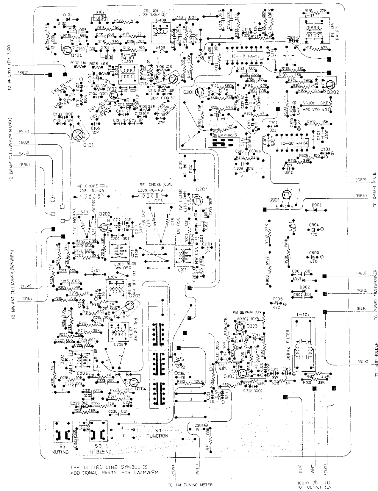
AM/FM/MPX Amp. Circuit Board Diagram (RT-425) Schaltbild des AM/UKW/MPX Verstärkers und Vorverstärkers (RT-425) Diagramme de Plaque du Circuit d'Amp. AM/FM/MPX (RT-425)
