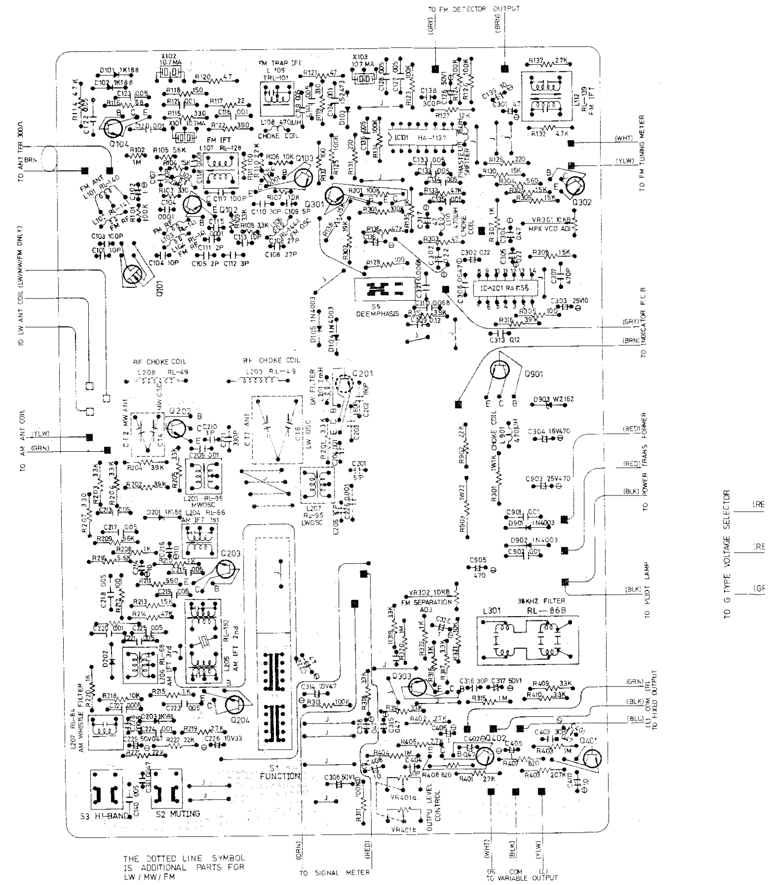
AM/FM/MPX Amp. Circuit Board Diagram (RT-725) Schaltbild des AM/UKW/MPX Vertärkers und Vorverstärkers (RT-725) Diagramme de Plaque du Circuit d'Amp. AM/FM/MPX (RT-725)
