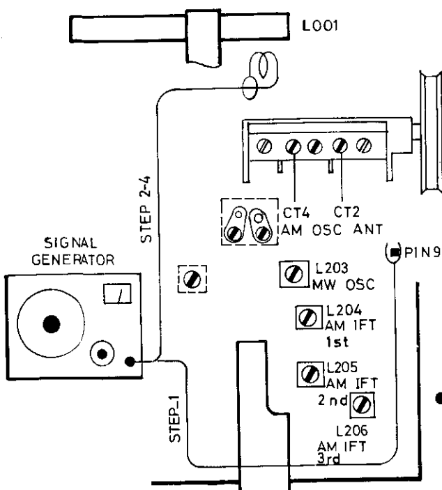
Fig. 1. AM IF and RF Alignment Hook-Up (RT 425) Abb. 1. AM-ZF und HF-Abgleich (RT 425) Fig. 1. Alignement AM IF et HF (RT 425)
