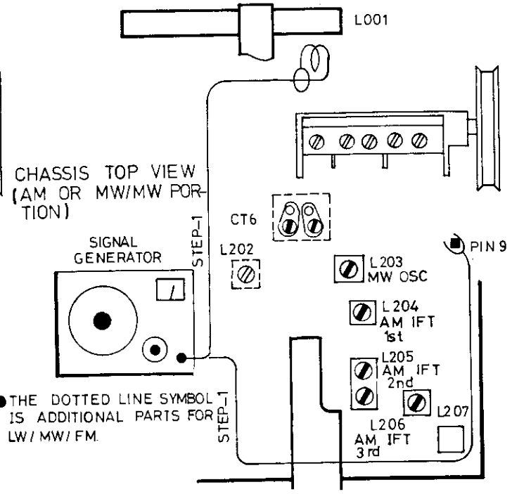
Fig. 2. AM IF and RF Alignment Hook-Up (RT 725) Abb. 2. AM-ZF und HF-Abgleich (RT 725) Fig. 2. Alignement AM IF et HF (RT 725)
