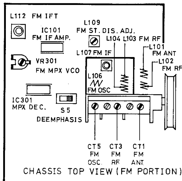
Fig. 4. FM IF and RF Alignment Hook-Up Abb. 4. UKW-ZF- und HF-Einstellung Fig. 4. Alignement FM IF et HF
