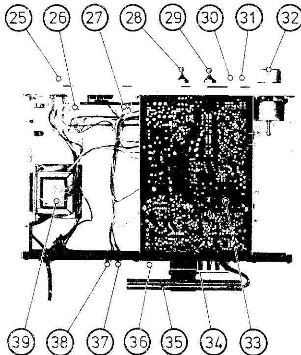
(Bottom View) (Unteransicht) (vue de dessous)
