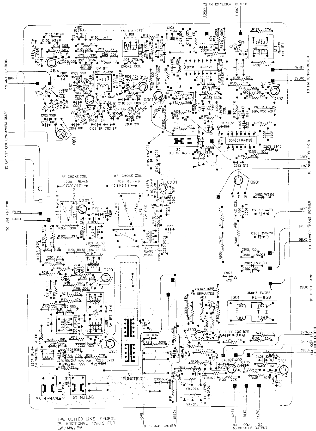
AM/FM/MPX Amp. Circuit Board Diagram (RT-725) Schaltbild des AM/UKW/MPX Vertaerkers und Vorverstaerkers (RT-725) Diagramme de Plaquette du Circuit d'Amp. AM/FM/MPX (RT-725)
