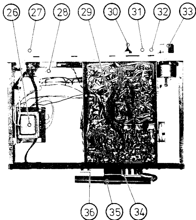
(Bottom View) (Unteransicht) (vue de dessous)
