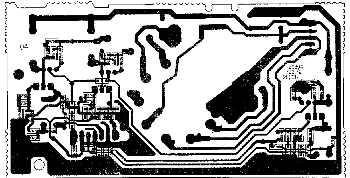
Chipbestückung, Ansicht auf die Lötseite Chip Components, view to the solder side
