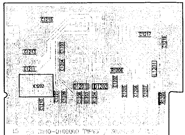
Chip-Seite/Chip view
