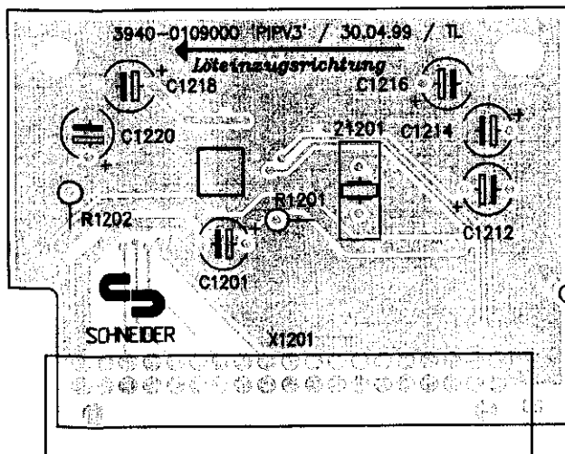
Bestückungsseite/Top view
