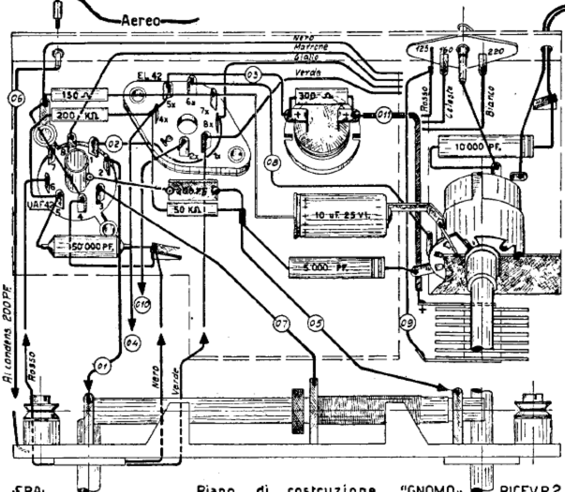
ERA Piano di costruzione "GNOMO" RICEV. R 2
