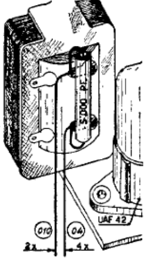
ERA Piano di costruzione "GNOMO" RICEV. R 2
