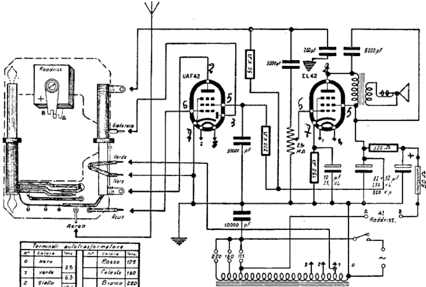
ERA Schema elettrico "GNOMO" RICEV. R 2
