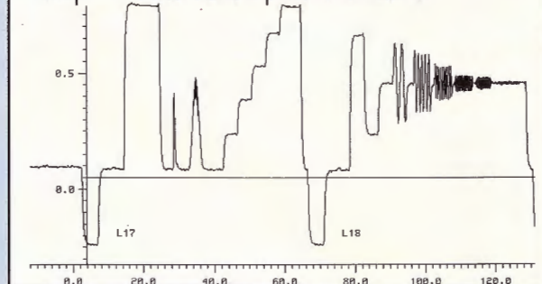
Réception avec bande passante réduite
