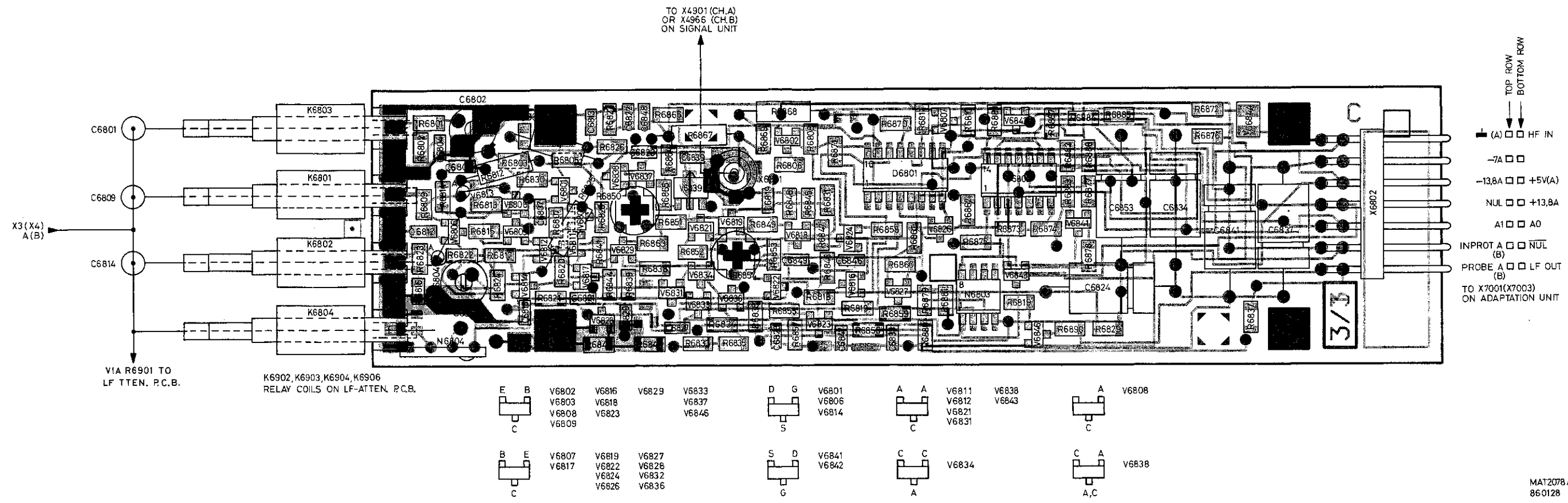
Fig.10.1. HF attenuator unit, p.c.b. lay-out.
