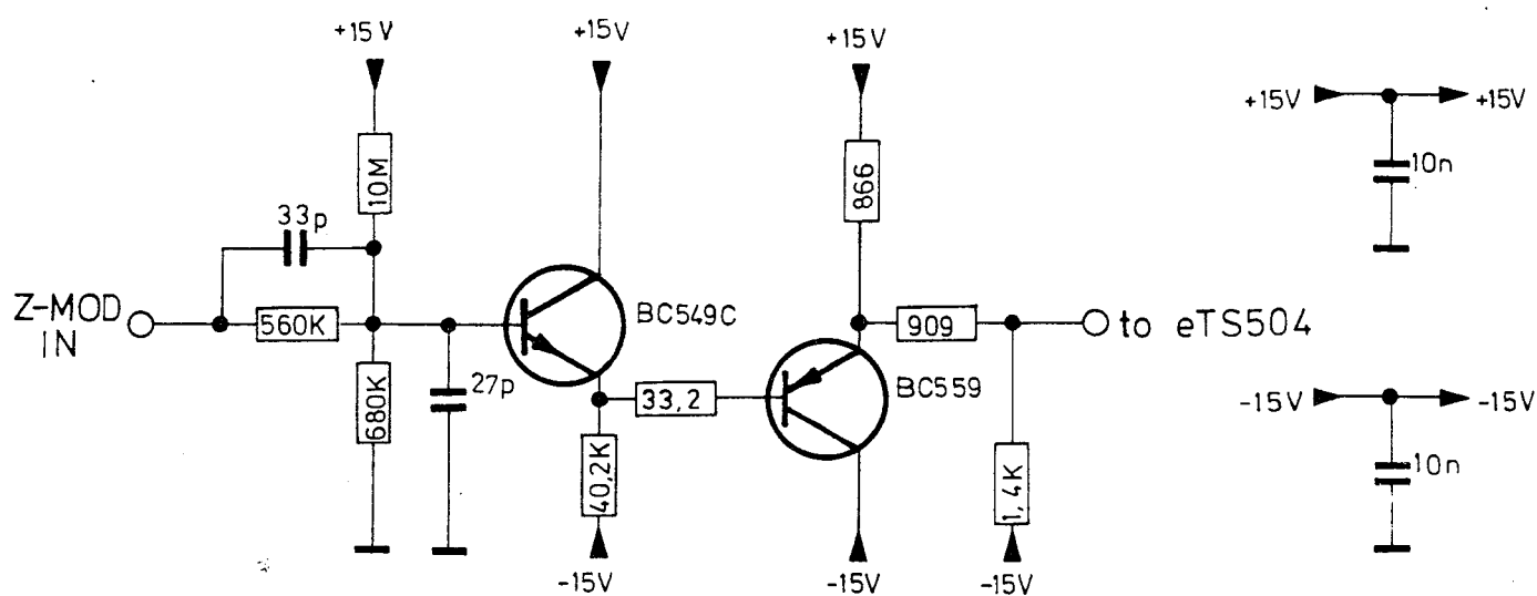
FIG.7 EXT. Z-MOD INPUT PM3260
