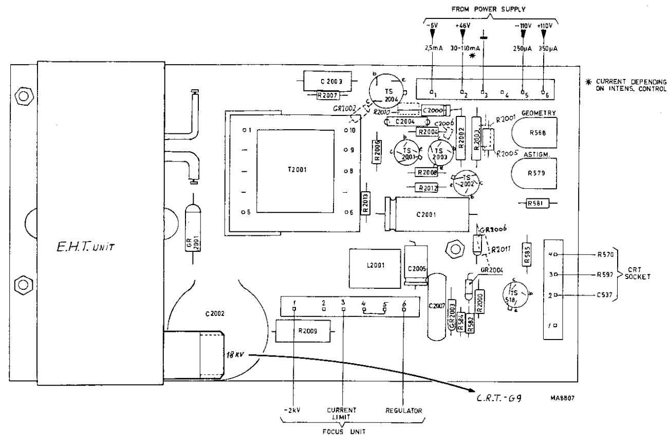
Fig. 3.63. 2 kV Unit
