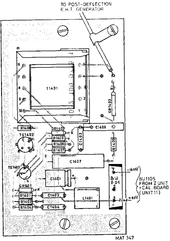
Fig. 3.39. E.H.T. converter p.c. board
