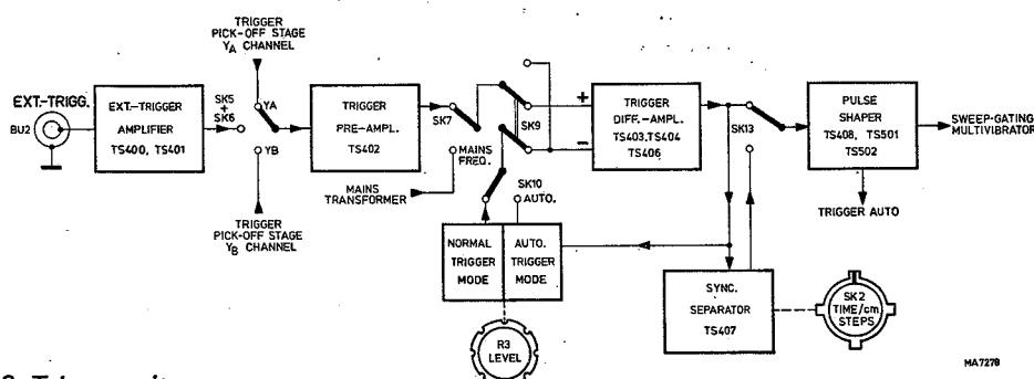
Fig. 3.3. Trigger unit
