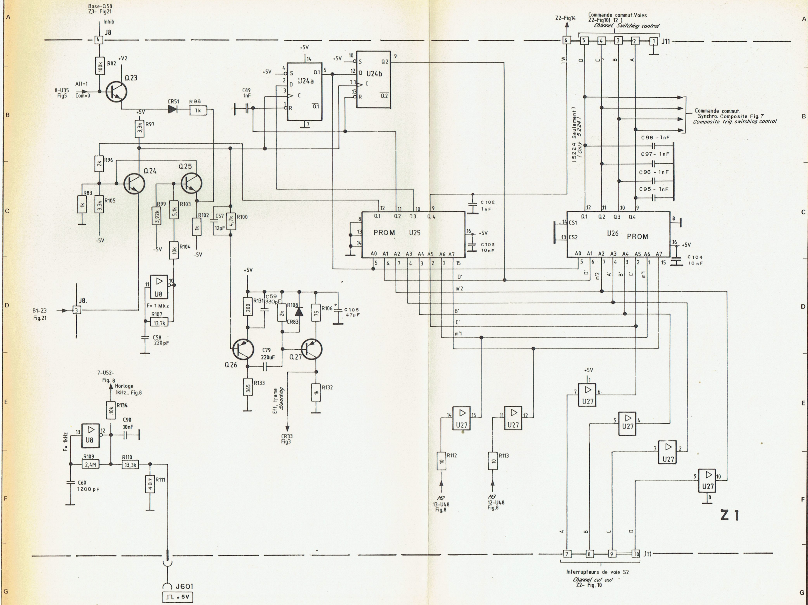
Fig 6 LOGIQUE Y
