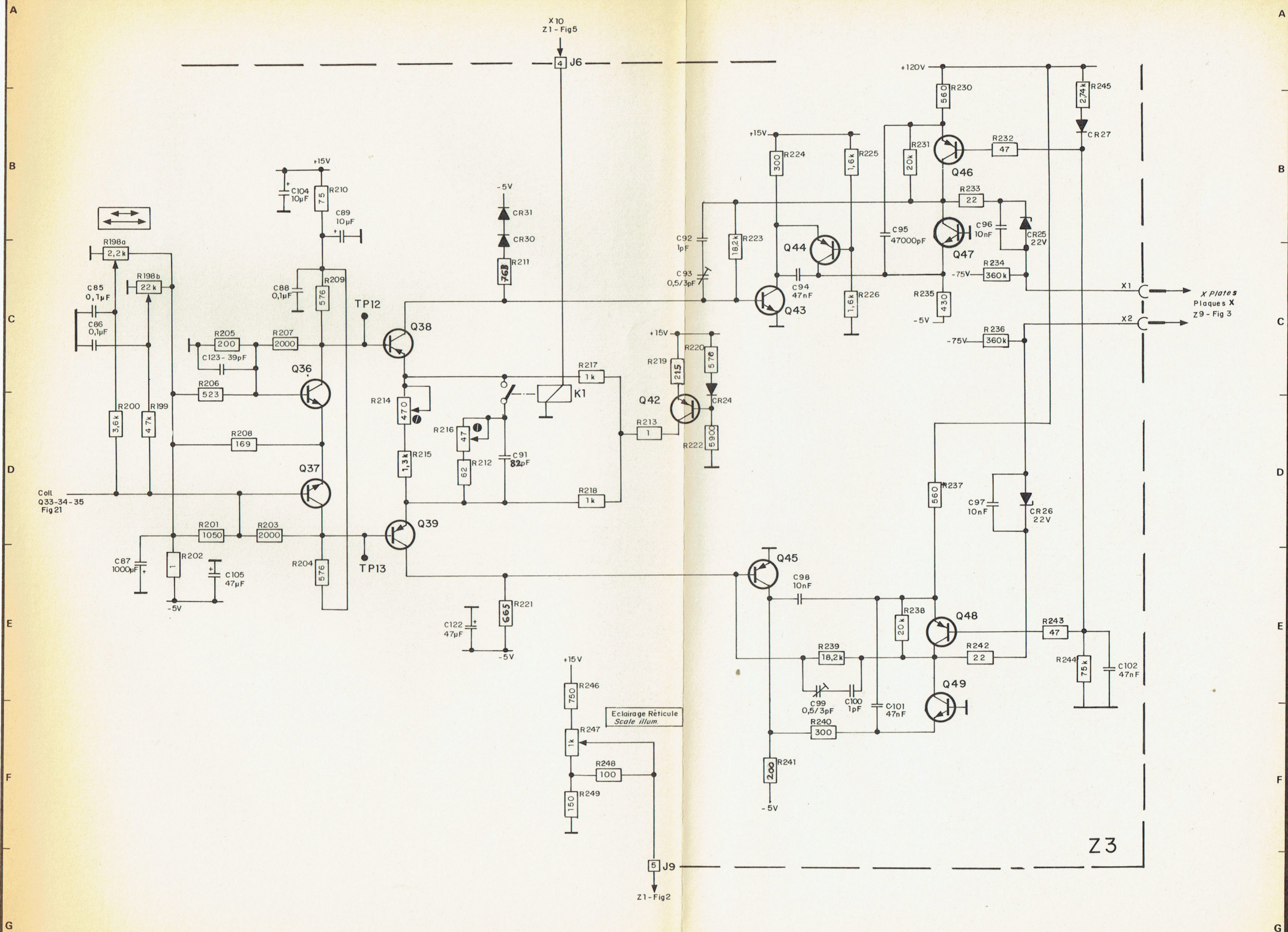
Fig 22 AMPLIFICATEUR HORIZONTAL HORIZONTAL AMPLIFIER
