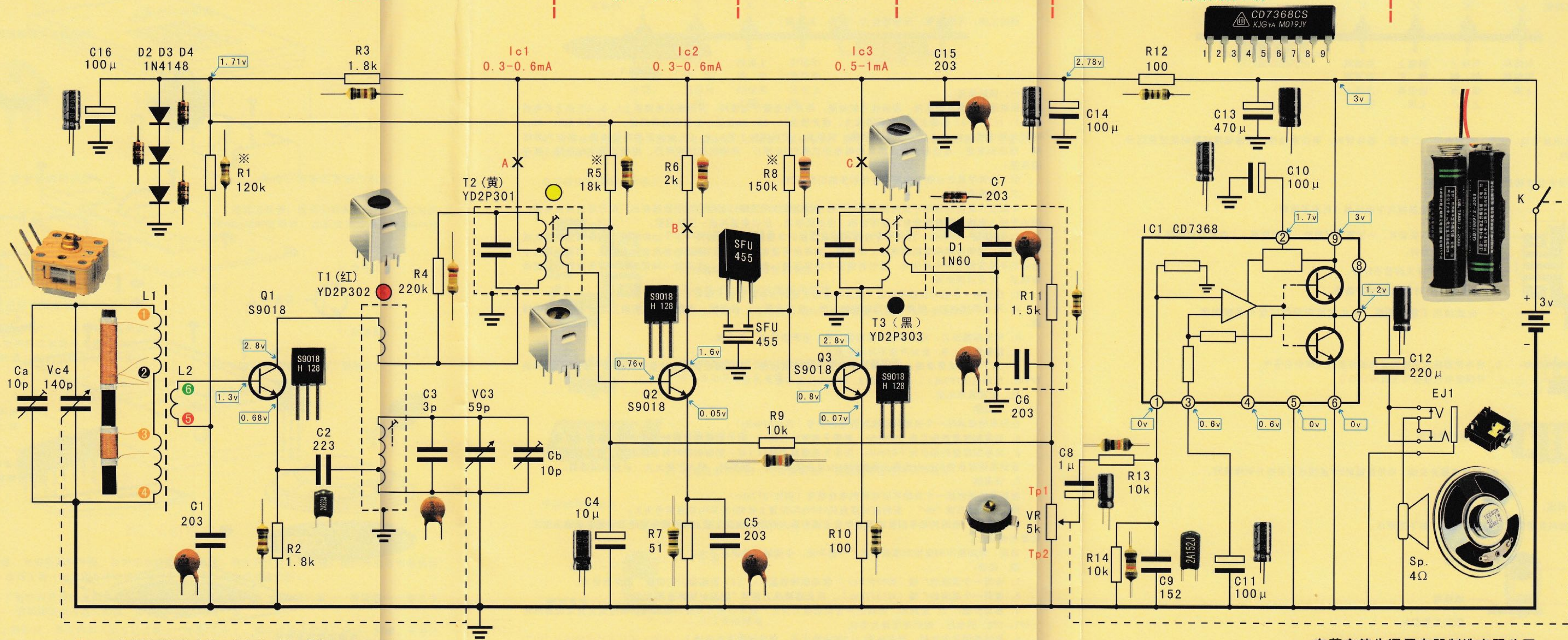
图5：“2P3”超外差式中波收音机电路图
