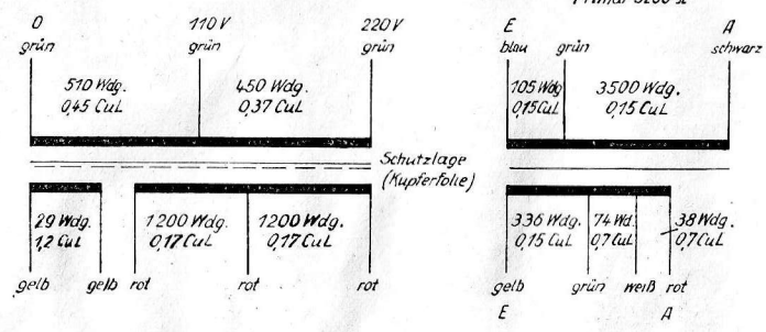
Netztransformator
