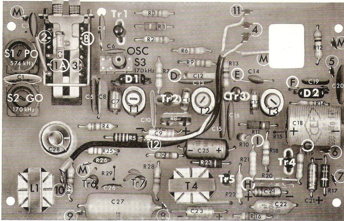
Circuit imprimé vu côté Cablage
