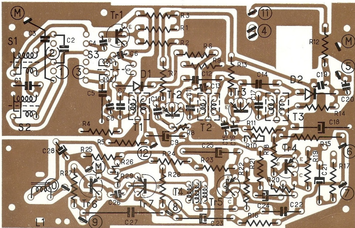
Circuit imprimé vu côté Cablage
