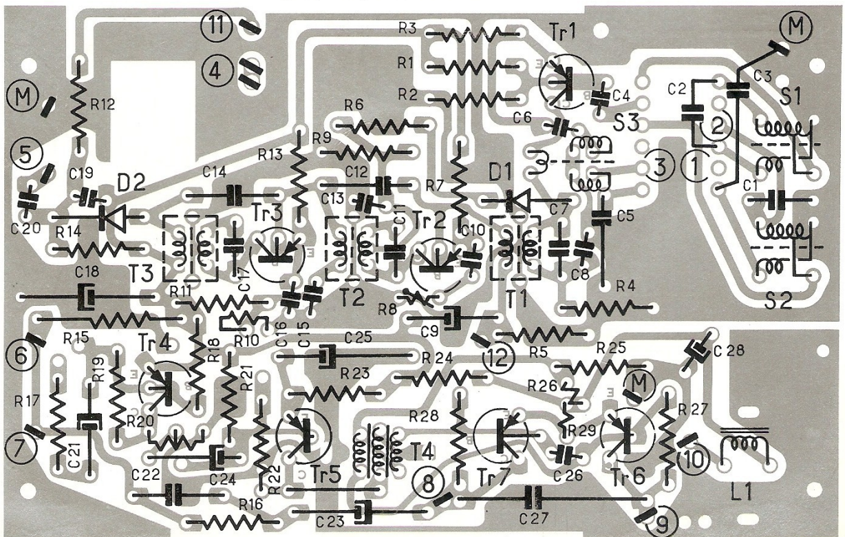
Circuit imprimé vu côté Soudure
