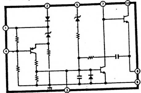
IC650 [STK7348]
