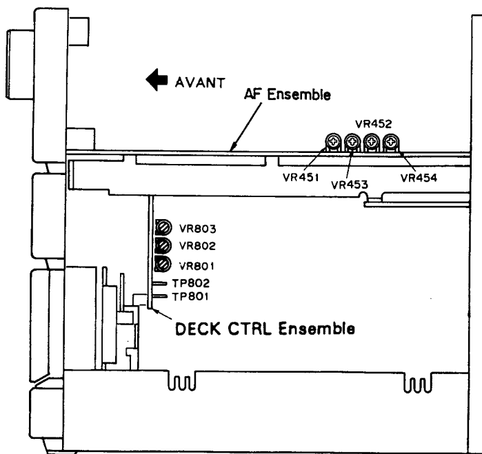
Fig 6.2 Points de réglage
