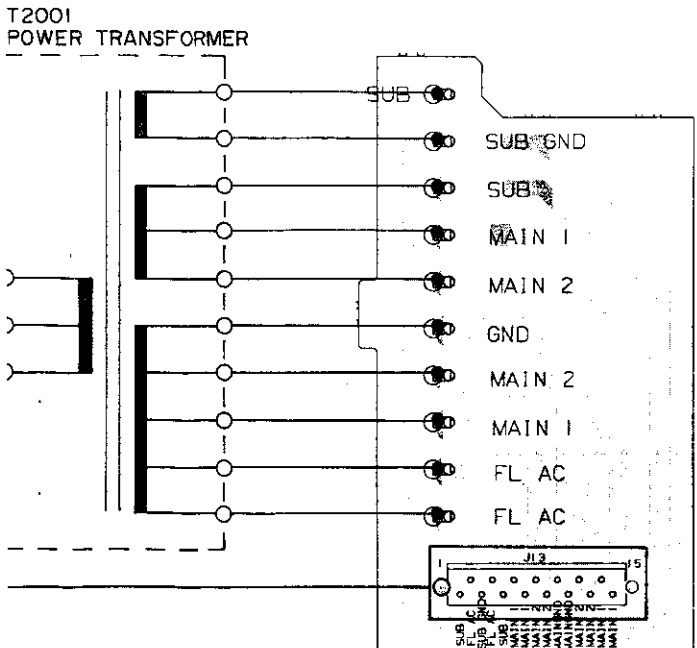
TRANS CONNECT assembly yldmegg T2ART
