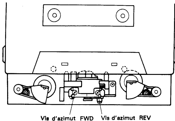
Fig. 6.4 Réglage d'azimut de la tête
