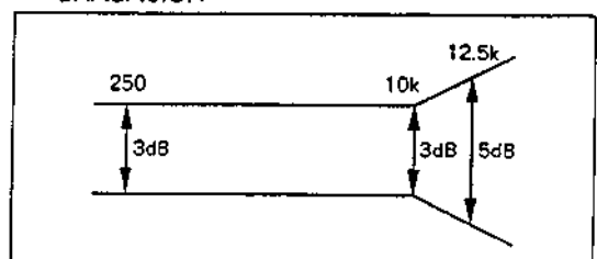
Figura 8-5 Zona de respuesta de frecuencia
