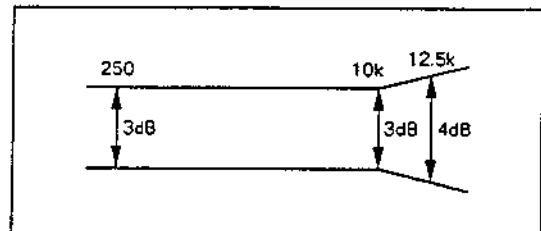
Figura 8-3 Constantes de la cinta de prueba STD-331E
