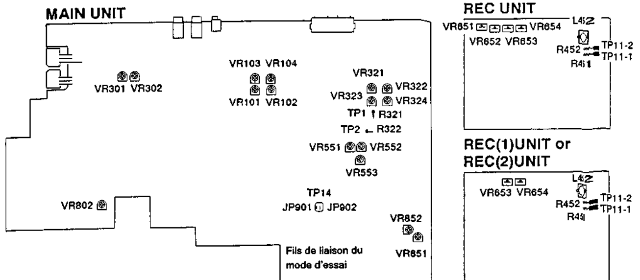
Fig. 8-2 Points réglage
