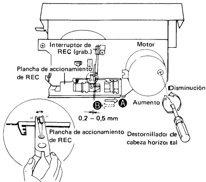
Fig. 11-2 Ajuste de la velocidad de la cinta y del interruptor de grabación (REC)
