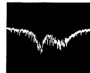
Fig. 9. 455 kHz trap.
