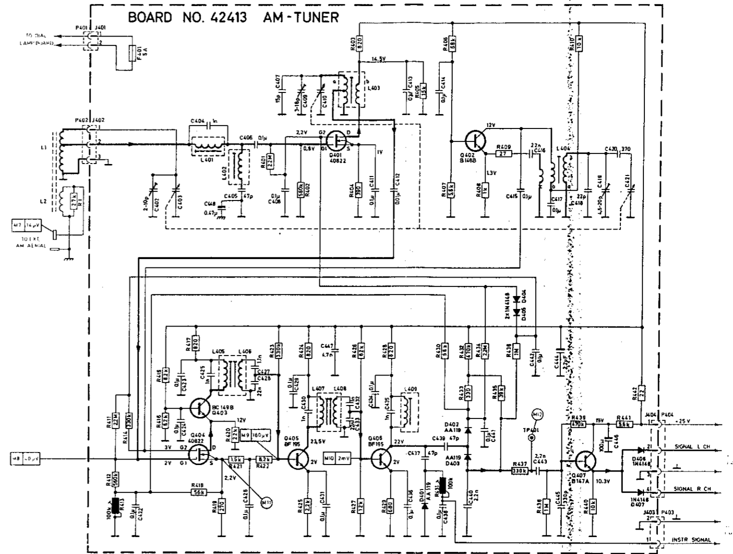
AM-SECTION - 42599
