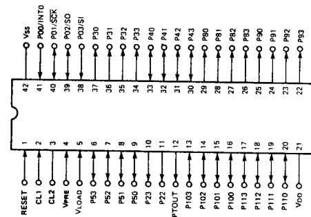
IC 607, 801: \mu PD7538
