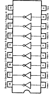
IC619, 620, 803: AN6873
