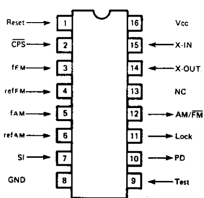
IC4: M54927P (Tuner Circuit)
