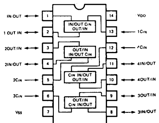
IC601, 602: M4066BP
