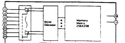
IC7701 HM6264ALSP
