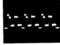
⑥3.6Vp-p(H)
