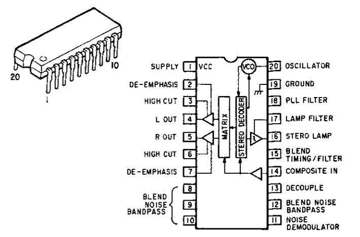
ULH3827A
