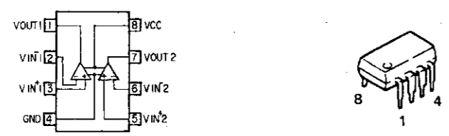
NJM4558D-D
