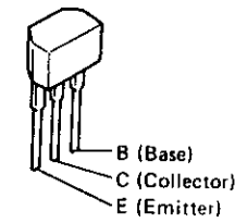
2SA1048(Y/GR) 2SC2458(Y/GR)
