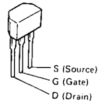
(FET) 2SK365(BL/GR)
