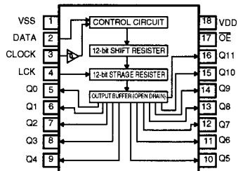
BU2090F (IC302, 602)
