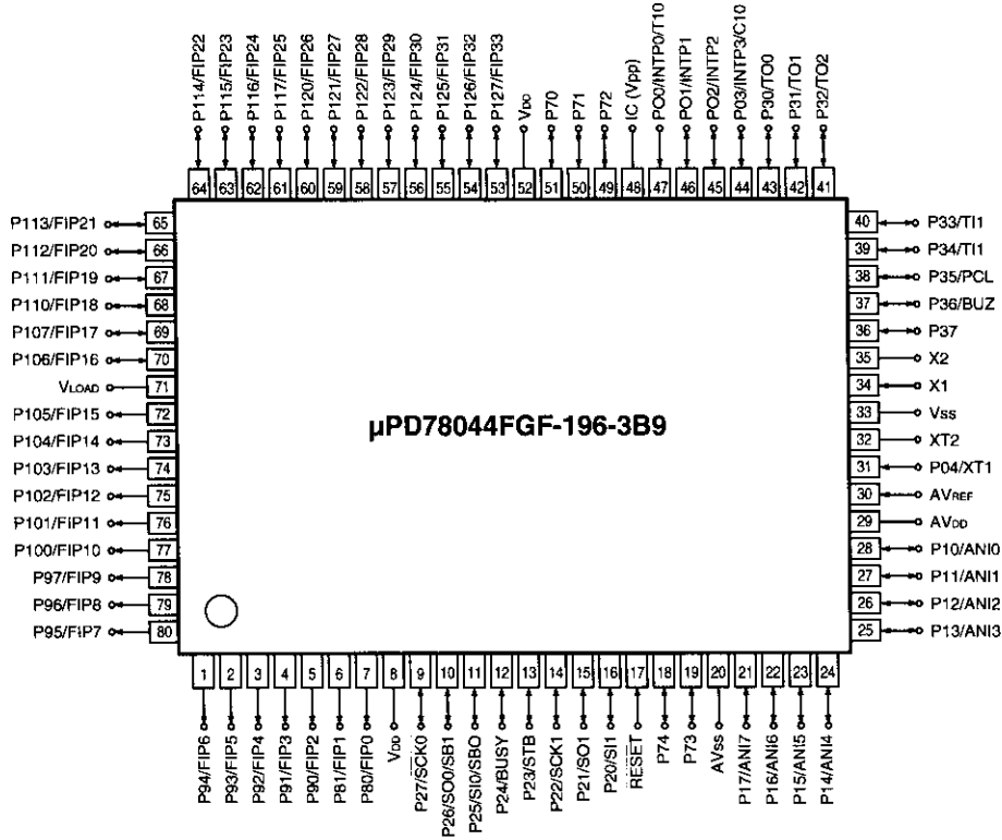
μPD78044FGF-196-3B9 Terminal Function
