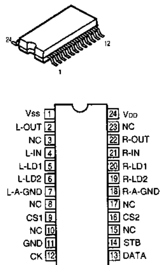
KIC9459F (IC111)
