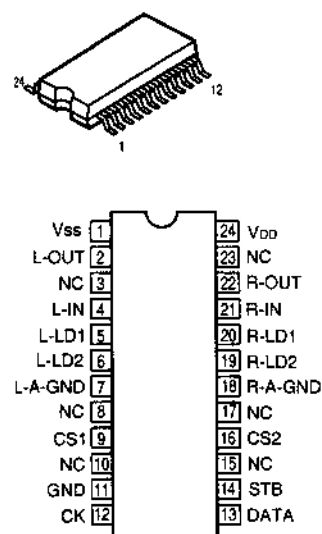
KIC9459F (IC111)
