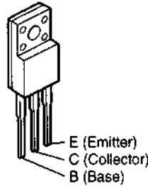
KTD2058
