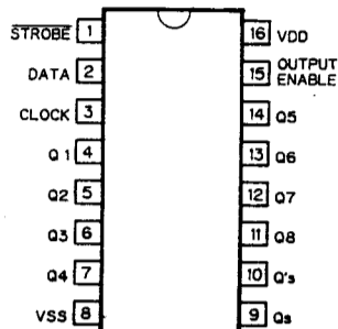
μPD4094BC
