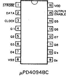
μPD4094BC
