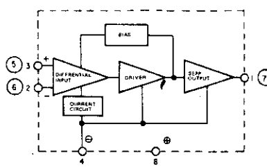
M54565P (Mitsubishi)
