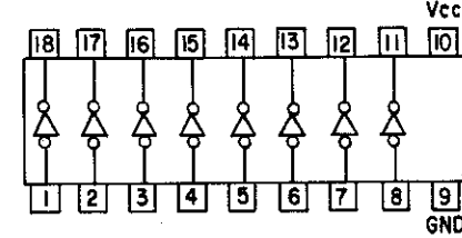
M54565P (Mitsubishi)
