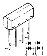
UB-152LFA
