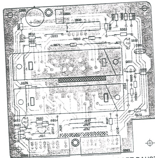
DOUBLE SCART BOARD / DOPPEL - SCART BAUSTEIN / CIRCUIT IMPRIME DE LA DOUBLE PRISE PERITELLE
