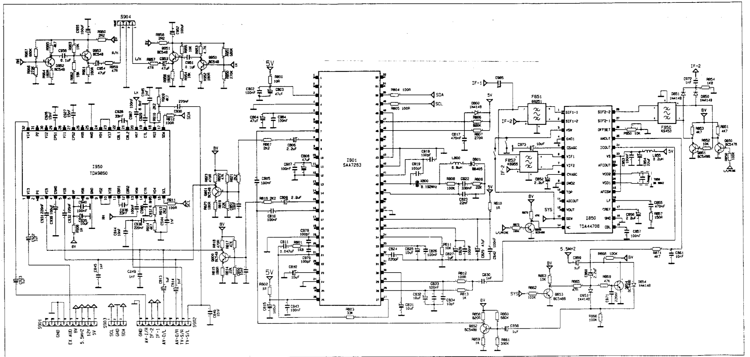
PT2 NICAM L BOARD CIRCUIT DIAGRAM / PT2 NICAM L BAUSTEIN SCHALTUNGSPLAN / SCHEMA DU CIRCUIT NICAM L
