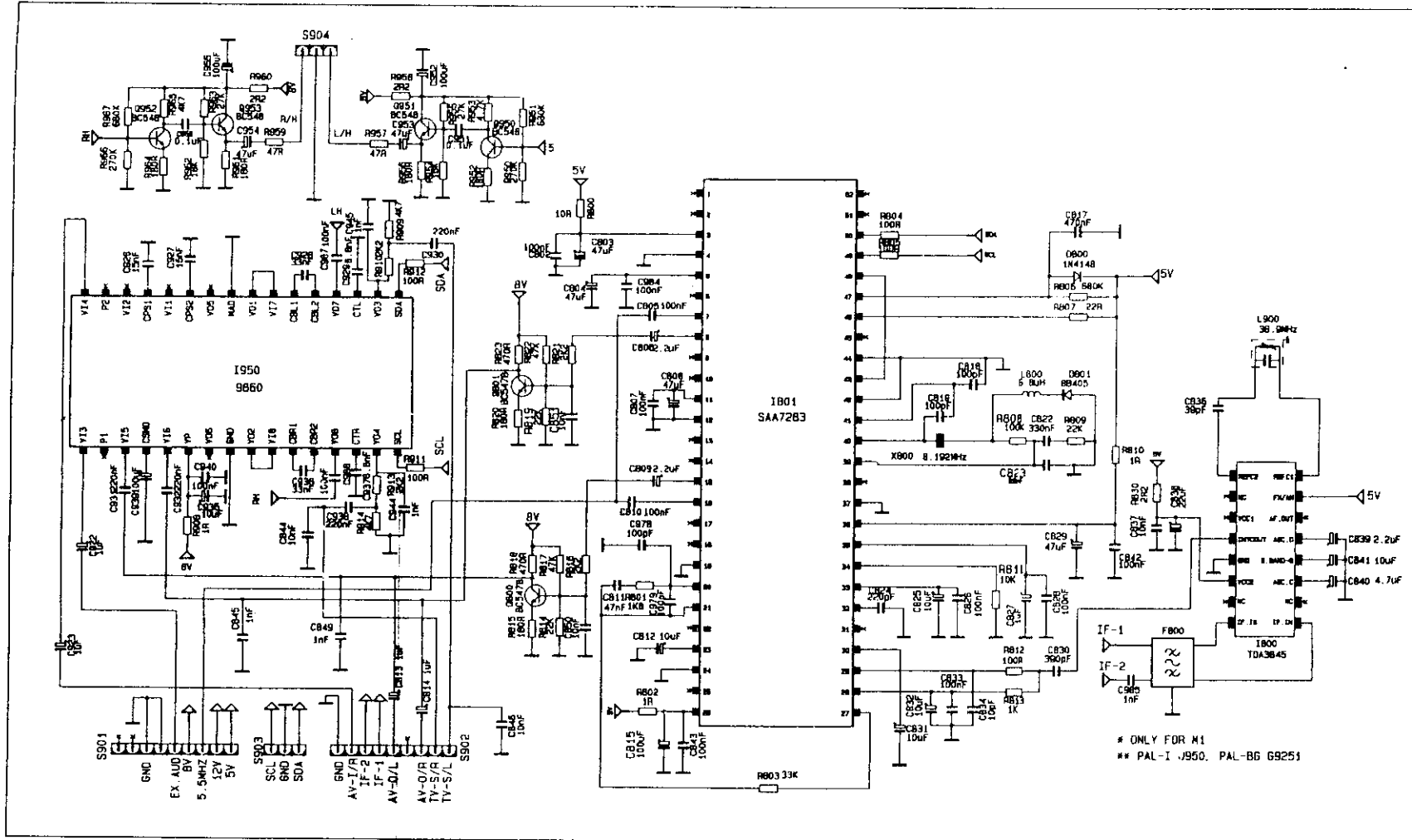
PT2 NICAM STEREO BOARD CIRCUIT DIAGRAM / PT2 NICAM STEREO BAUSTEIN SCHALTUNGSPLAN / SCHEMA DU CIRCUIT NICAM STEREO
