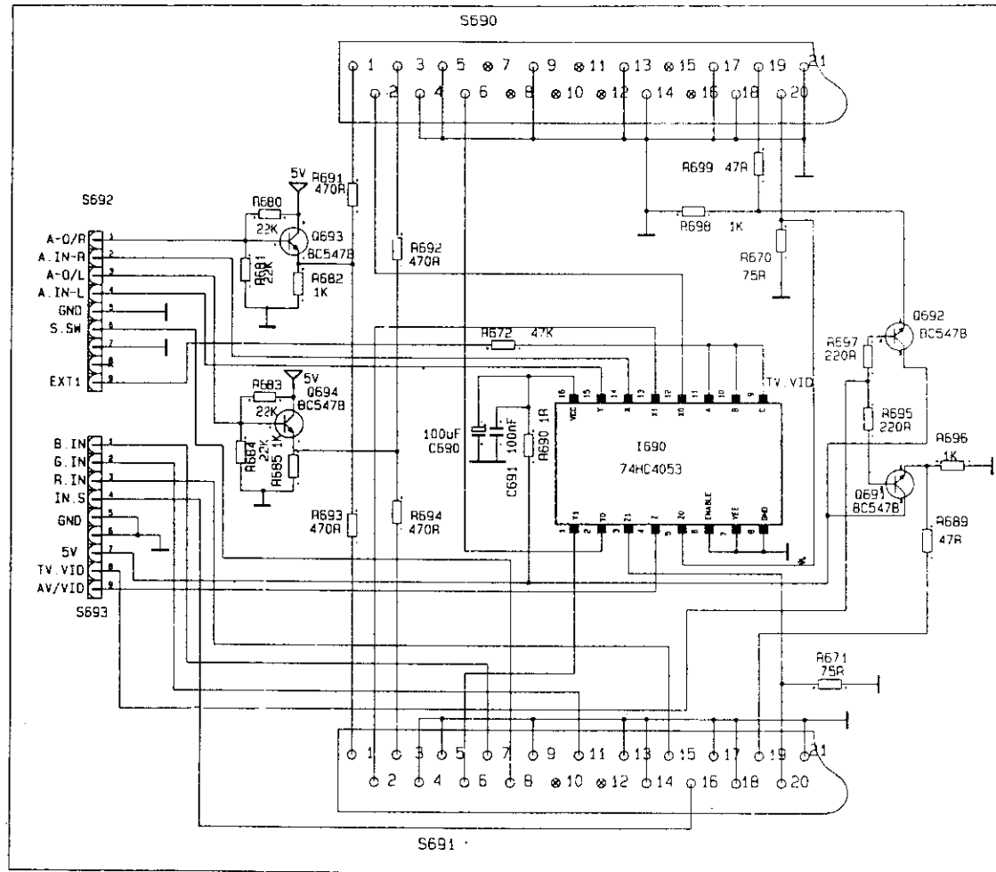
DOUBLE SCART BOARD CIRCUIT DIAGRAM / DOPPEL - SCART BAUSTEIN SCHALTUNGSPLAN / SCHEMA DU CIRCUIT DE LA DOUBLE PRISE PERITELLE
