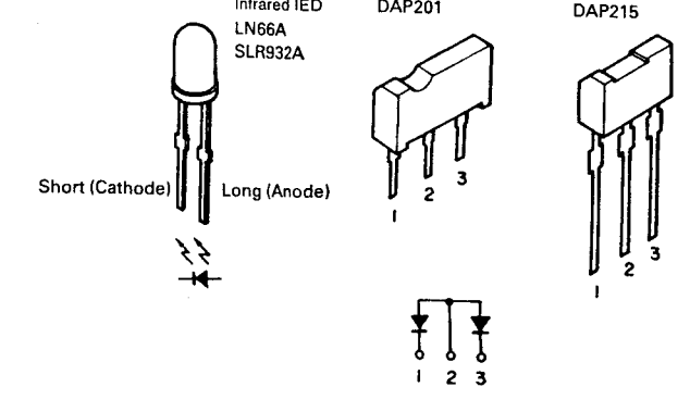
Diodes
