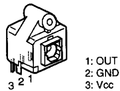
TOTX178A (IC601)
